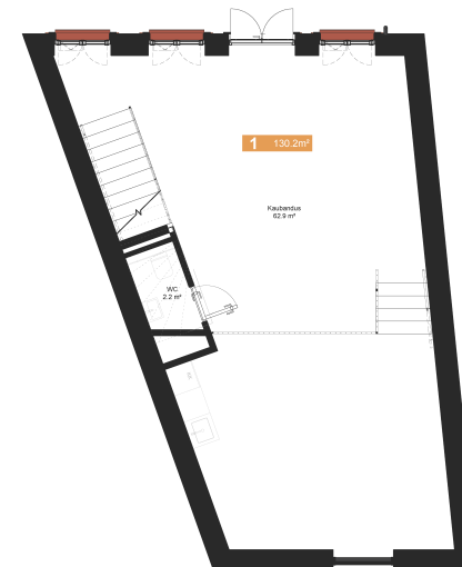
1. KORRUS
